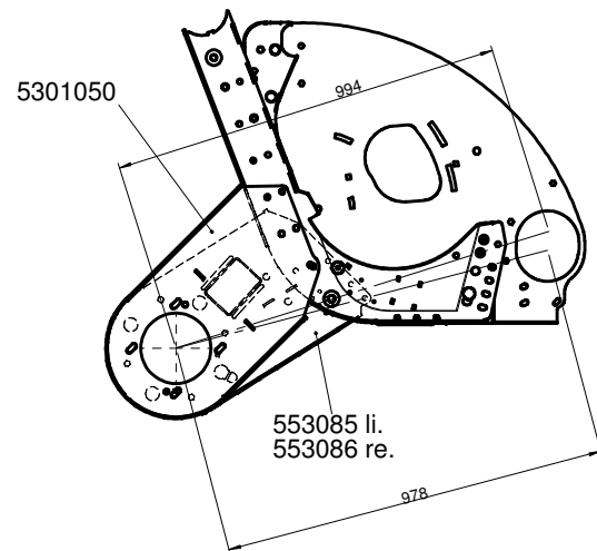
ATP 56v Lagerhalter 125mm verkröpft 5301130 re 5301131 li
