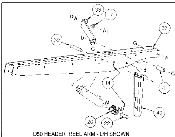
D50 HEADER REEL ARM - L/H SHOWN
